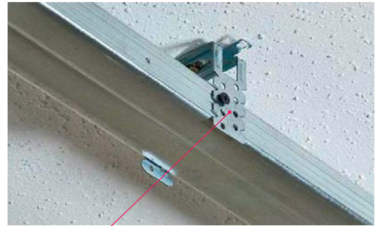
Direktabhängen für CD- Deckenprofile
